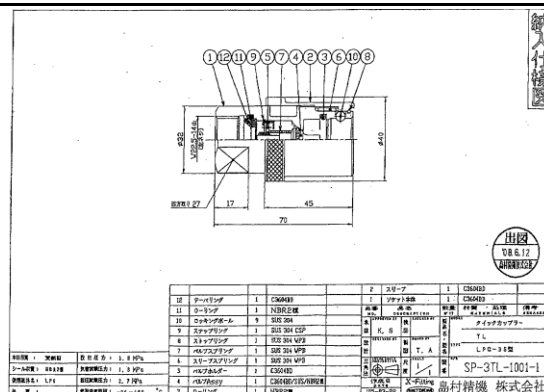
S 9 TL、TL-HX クイックカップ ラー兼用Oリング
